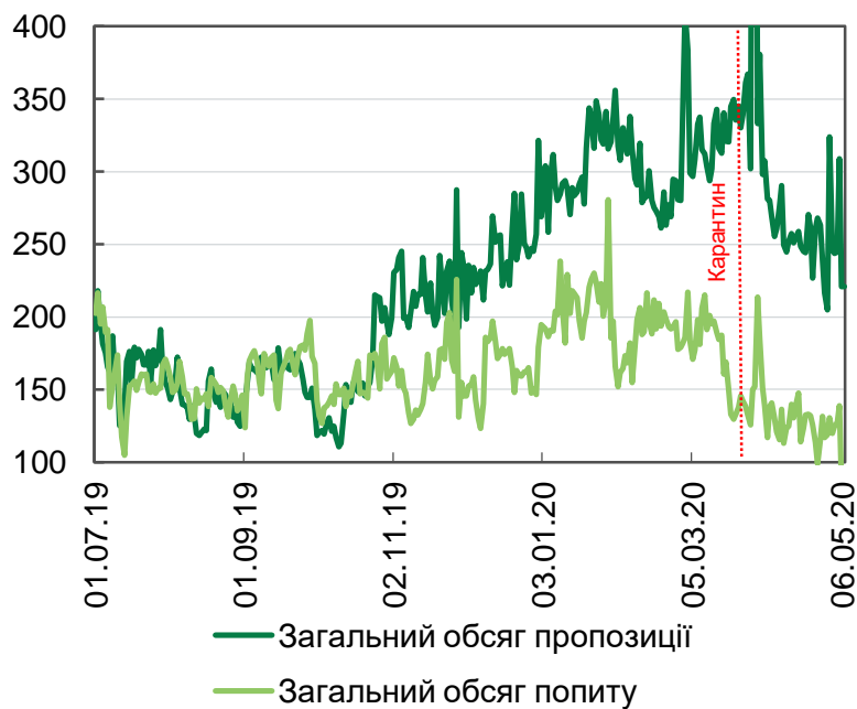
Обсяги попиту-пропозиції електроенергії на РДН/ВДР, ГВт-год
