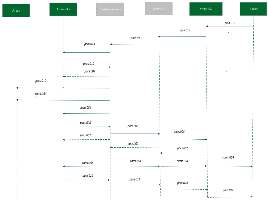
Рисунок 29. Функціональна схема
